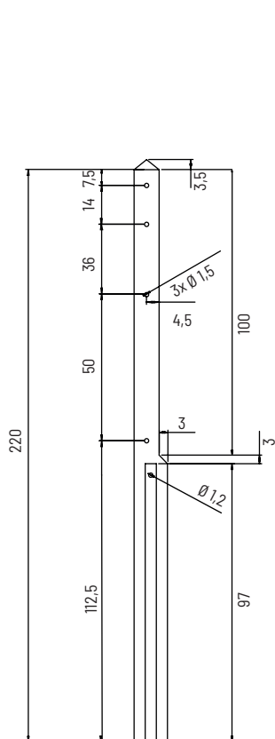
Poteau hauteur 2,20 m
