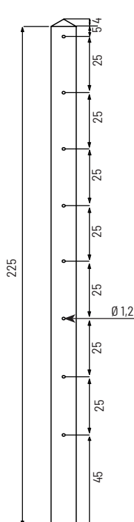
Poteau sans encoche
