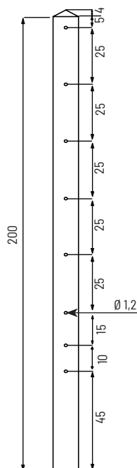
Poteau sans encoche
