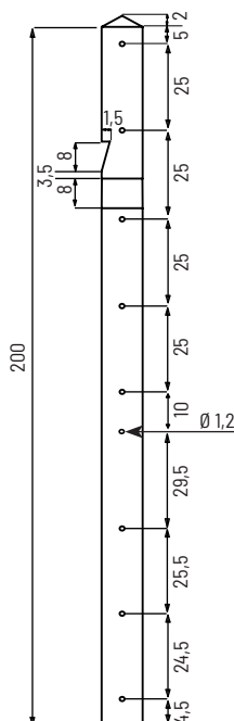
Poteau avec encoches / 3D
