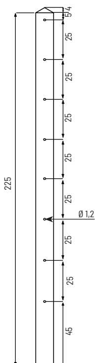
Poteau sans encoche
