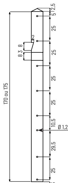
Poteau avec encoches / 3D
